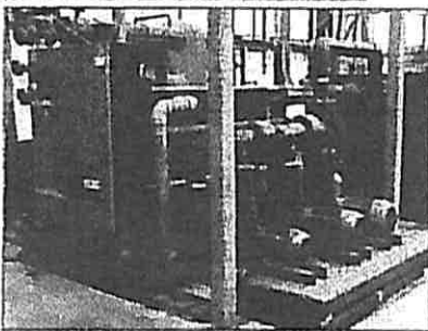
BERG 50 TON CHILLER MODEL WZ-50-2/1
